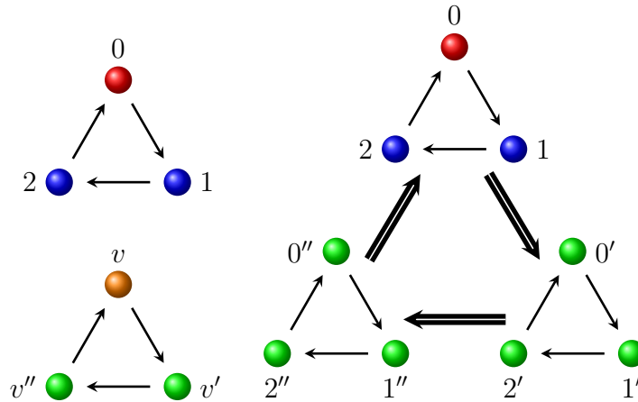
Figura 1.3: El torneo \vec{C}_3[\vec{C}_3] y una coloración heredada.
