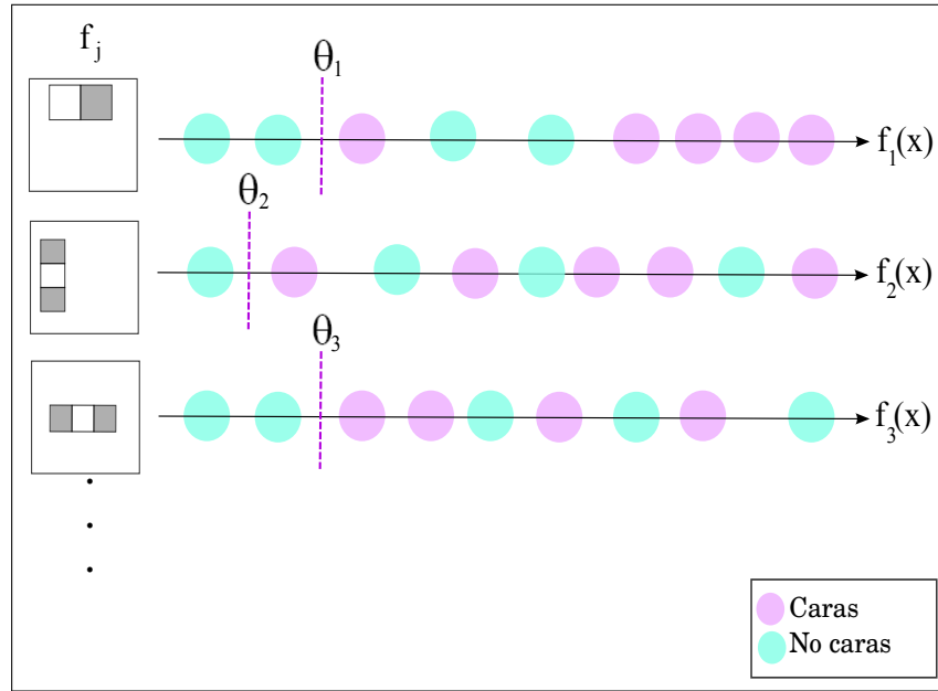
Figura 2.12: Creación de características débiles h_j
