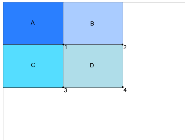
Figura 2.9: Cálculo de un área rectangular mediante imágenes integrales
