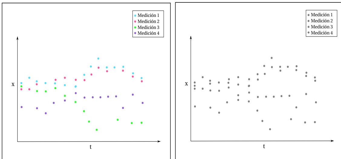
Figura 3.3: Multi-tracking con filtro de Kalman. Izquierda . Trayectorias clasificadas por objeto. Derecha . Trayectorias sin clasificar.
