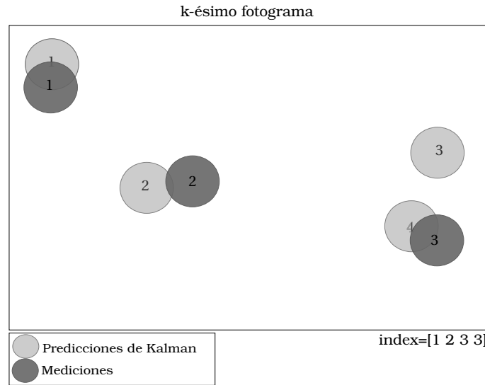
Figura 3.4: Asociación predicción-medición para la desaparición de objetos en la escena.
