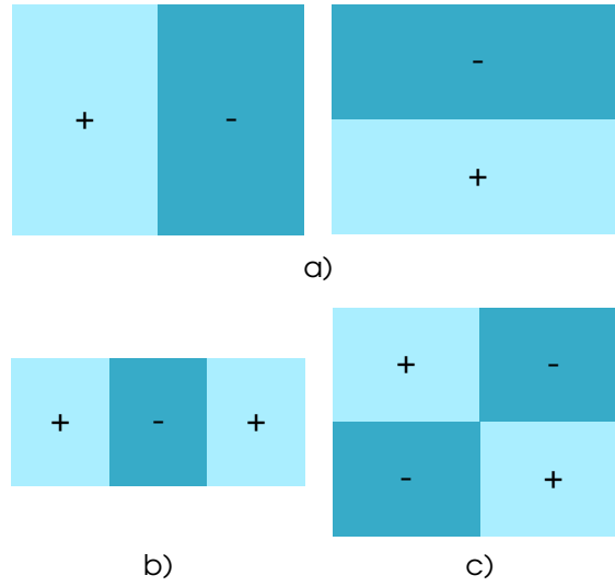
Figura 2.10: Características utilizadas en el método de Viola-Jones. a) two-rectangle. b) three-rectangle. c) four-rectangle
