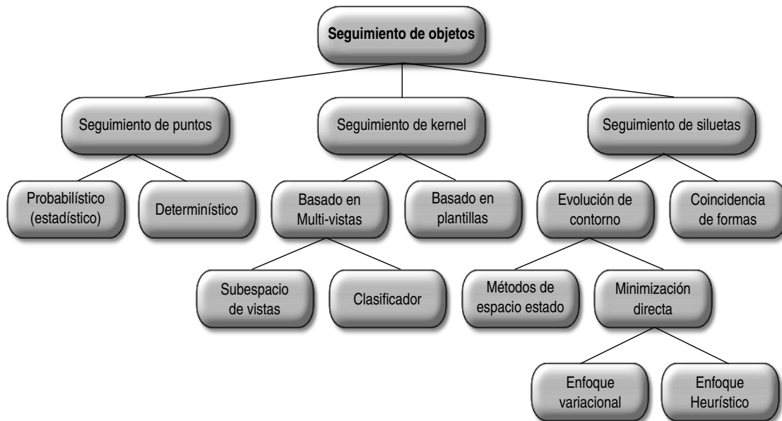
Figura 3.1: Taxonomía de los métodos de seguimiento de objetos. Yilmaz et al. [4].
