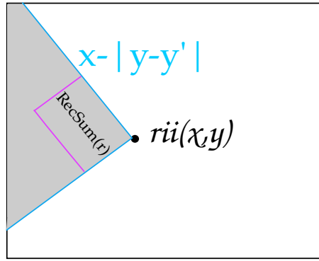
Figura 2.17: Cálculo de imagen integral y rectángulo rotado 135^\circ . R. y J. [3].
