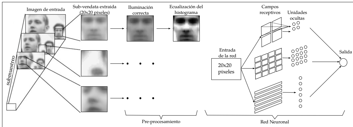
Figura 2.6: Proceso de detección de rostros de Rowley et al. [2].
